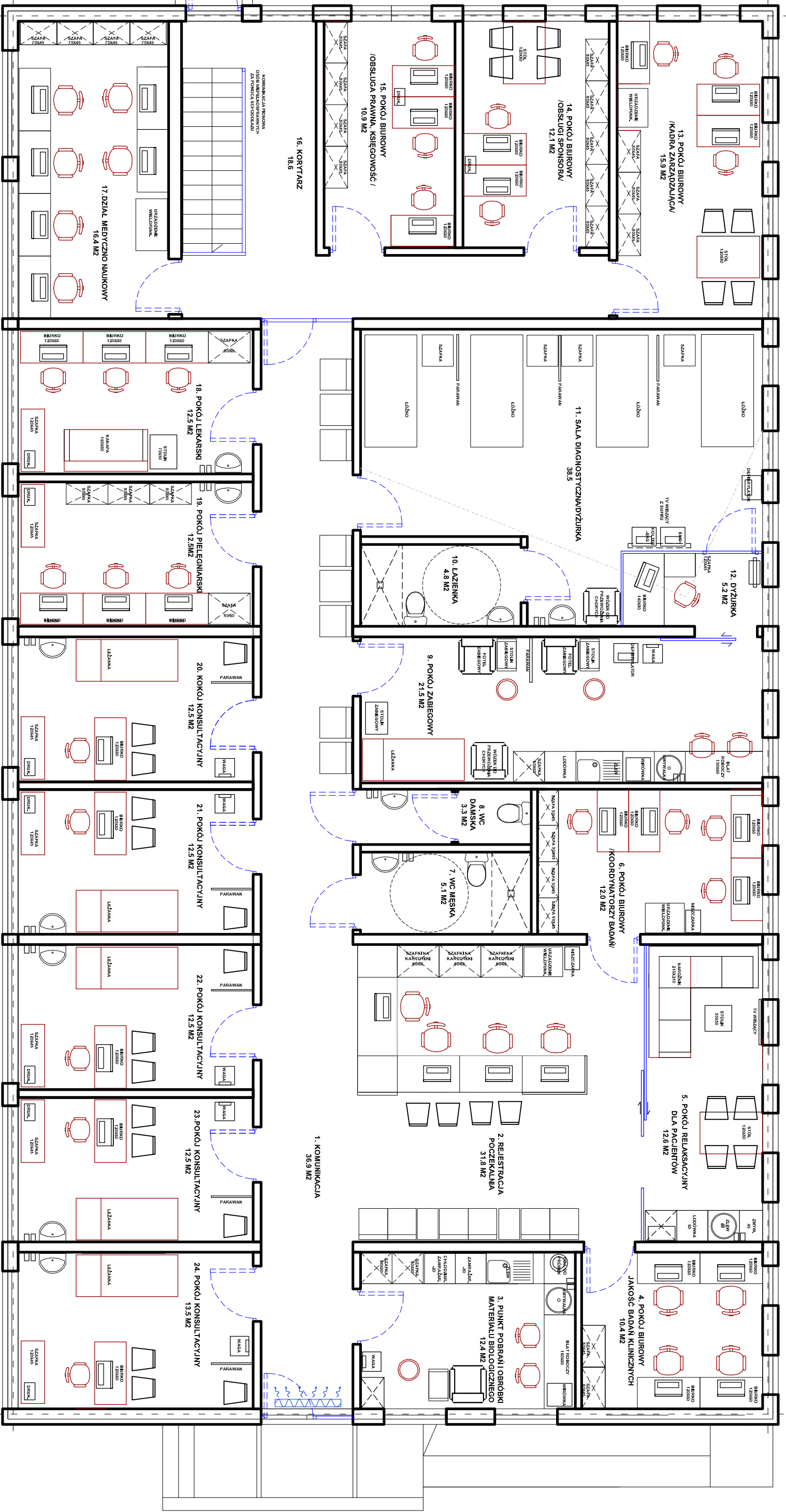
POZIOM 0 /UKŁAD FUNKCJONALNY/
